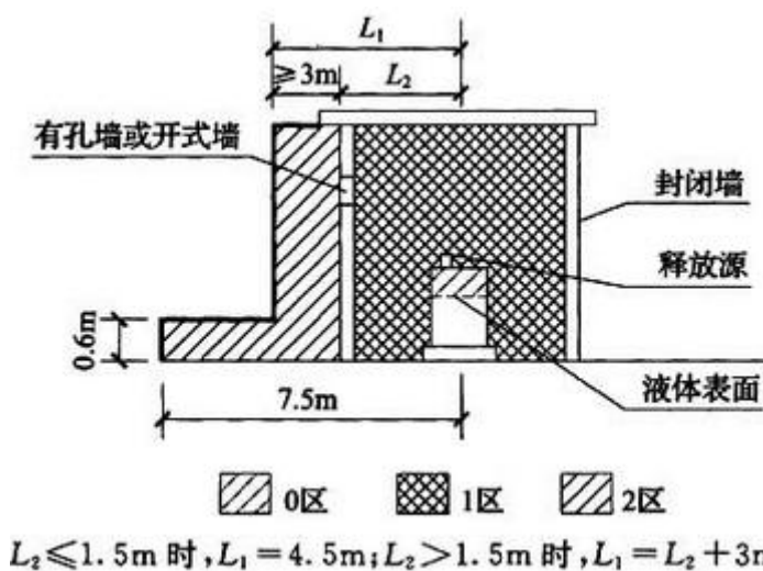
图 B.0.10 易燃液体灌桶间爆炸危险区域划分
